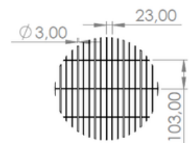
DETALHE ESCALA 2 : 25
